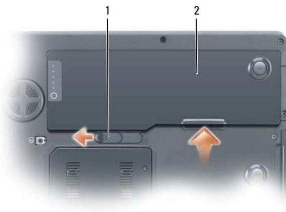
1 Akkufachfreigabevorrichtung 2 Akku
